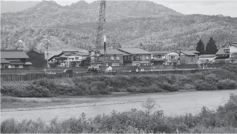
堤防の漏水対策工事の様子（来迎寺地区）
