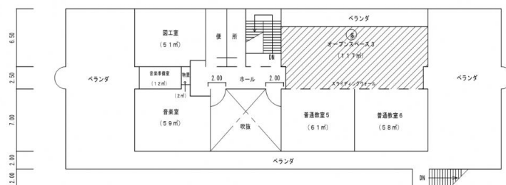
3 階 平 面 図 ⑧
