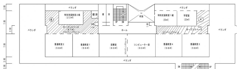
2 階 平 面 図 ⑧
